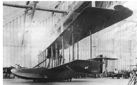
Hydravion Curtiss HS-2L (1918). Vue latérale montrant la forme de la coque et de la voilure.
