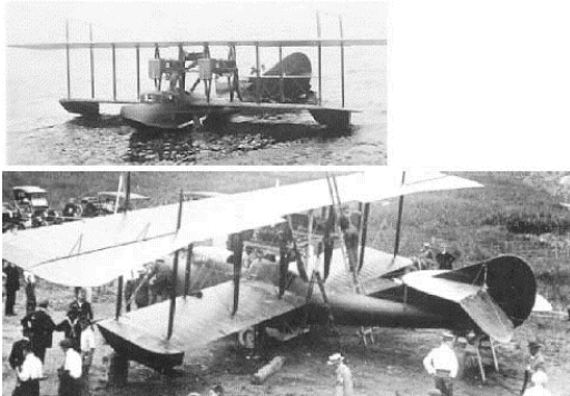
Hydravions américains Curtiss H-16, des appareils apparus en 1914 destinés à la formation des pilotes d'observation de l'U.S. Navy.
