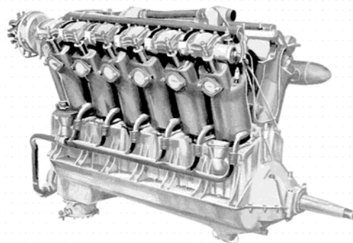
Moteur V12 Liberty de 400 ch (1918). V12 à 45° de 127 mm d'alésage et de 177 mm de course, cette mécanique utilisait volontairement une technologie simple pour faciliter sa maintenance.
